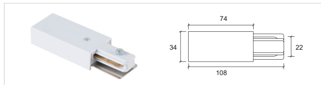
2 线直连接器 6201-I I - connector
