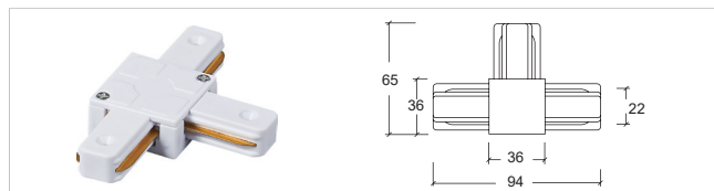
2 线三向连接器 6202-T T - connector
