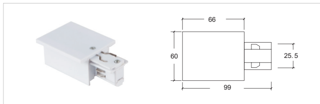
H-03 电源接驳器 - 左 Feeder-L
