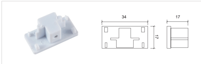
3 线 A 电源终接 End cap
