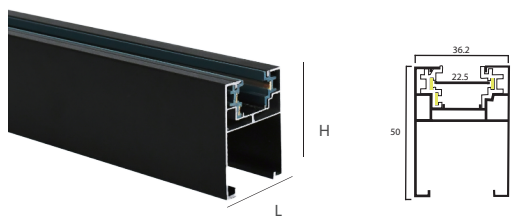
三线桥架电源头前插 feeder YZ6306-Q
