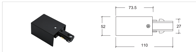
三线无缝i接 MINI Connector YZ6309-MI
