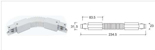
H-04 多角度接駁器 (软接) Flexible Connector
