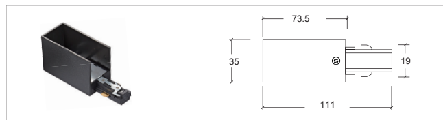
三线桥架外I接 Connector YZ6306-I
