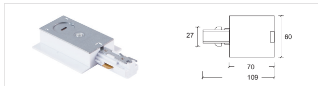
3 线 A 嵌入式直线接驳器 Straight connector
