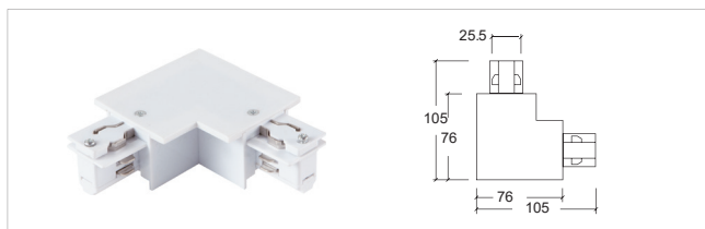
H-03 L型接驳器 - 左 L- connector - L
