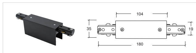
三线无缝1接 MINI Connector YZ6306-MI
