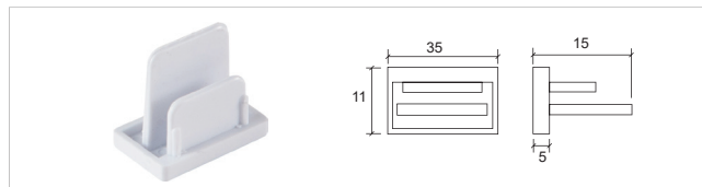
2 线 L 型连接器 6201-L L - connector
