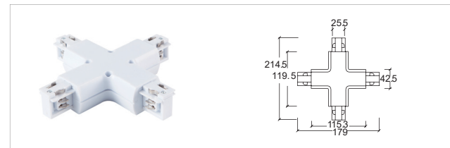
H-01 四向接驳器 X- connector
