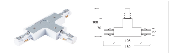
3 线 A 三向接驳器 - 左 T-connector - L
