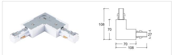
3 线 A L 型接驳器 - 左 L-connector - L
