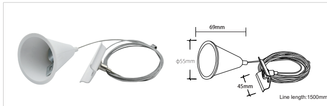
H-01 四线吊装线 Fitting
