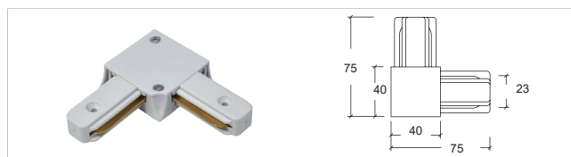
2 线 L 型连接器 6202-L L - connector
