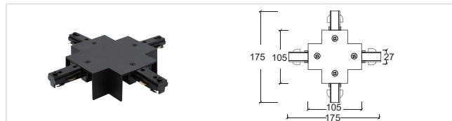
三线桥架外X接 X Connector YZ6317-X
