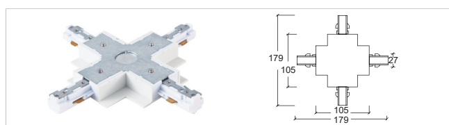
3 线 A 嵌入式四向接驳器 X-connector
