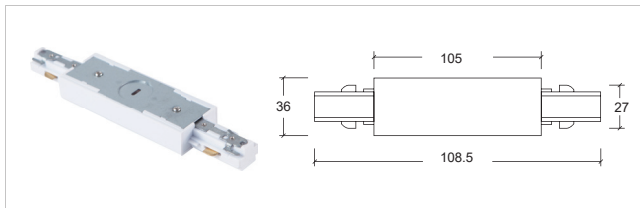
3 线 A 直线接驳器 Straight connector
