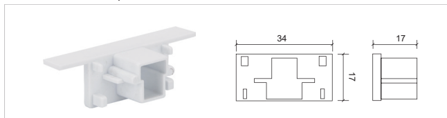
3 线 A 嵌入式 L 型接驳器 - 左 L-connector - L
