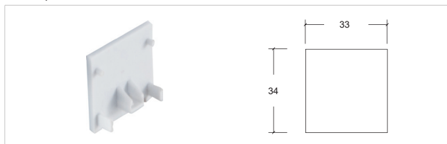
H-03 电源终接 End cap
