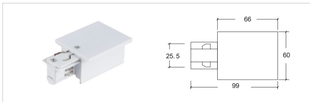
H-03 电源接驳器 - 右 Feeder-R
