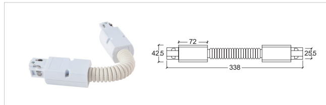
H-01 多角度接驳器 (软接) Flexible Connector
