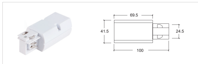
H-01 电源接驳器 - 左 Feeder-L
