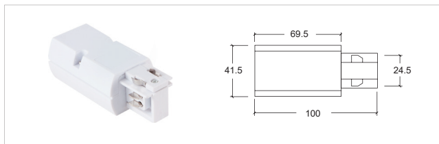
H-01 电源接驳器 - 右 Feeder-R
