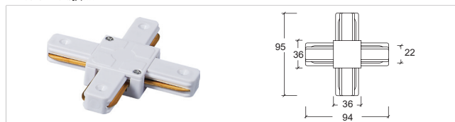
2 线四向连接器 6202-X X - connector
