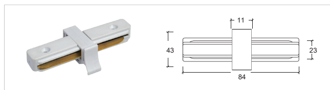
2 线直连接器 6202-I Straight connector
