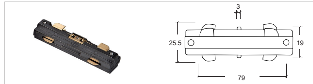
三线桥架外L接 L Connector YZ6317-L
