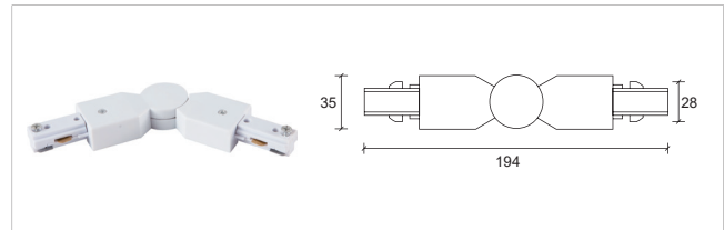
任意角度接驳器 Flexible Connector
