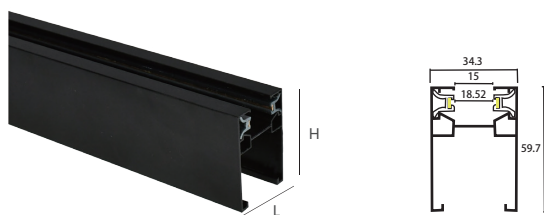
二线桥架电源头 Feeder YZ6216-Q
