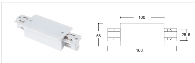
H-03 直线接驳器 Straight connector
