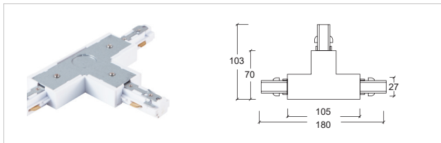
3 线 A 三向接驳器 - 右 T-connector - R
