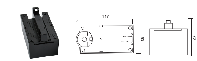
导轨盒-迷你盒Guide Box - Mini Box S036
