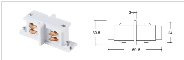
H-04 迷你型直线接駁器 Straight connector MINI
