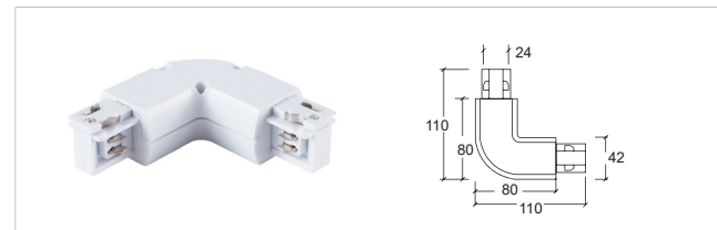
H-01 L型接驳器 - 右 L- connector - R
