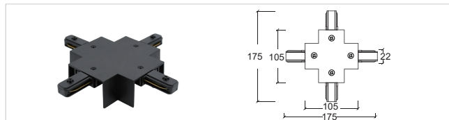
二线桥架外X接 X Connector YZ6222-X
