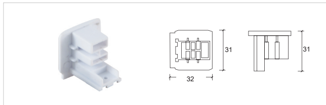
H-04 电源终接 End cap
