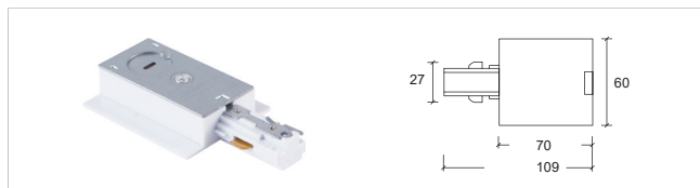
3 线 A 电源终接 End cap
