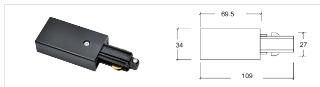
3 线 A 迷你型直线接驳器 YZ6313-Mini I Connector
