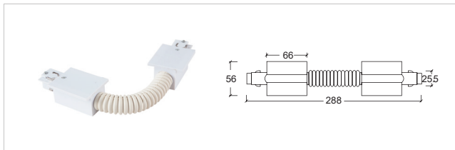
H-03 多角度接驳器 (软接) Flexible Connector
