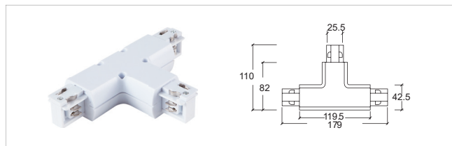
H-01 三向接驳器 - 右 T- connector - R
