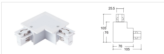
H-03 L型接驳器 - 右 L- connector - R
