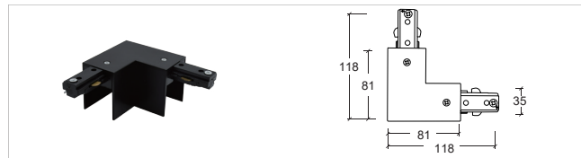
三线桥架外T接T Connector YZ6306-T
