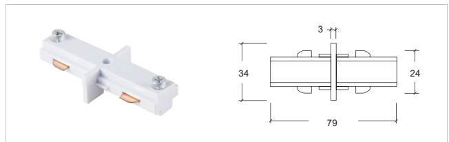
3 线 A 迷你型直线接驳器 Straight connector MINI
