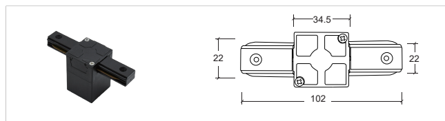
二线无缝1接 MINI Connector YZ6216-MI
