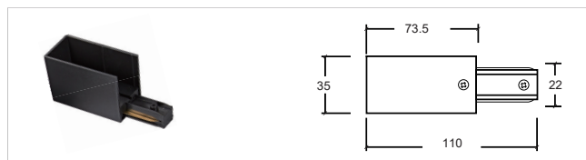
二线桥架外I接 Connector YZ6216-I
