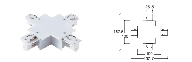
H-03 四向接驳器 X- connector
