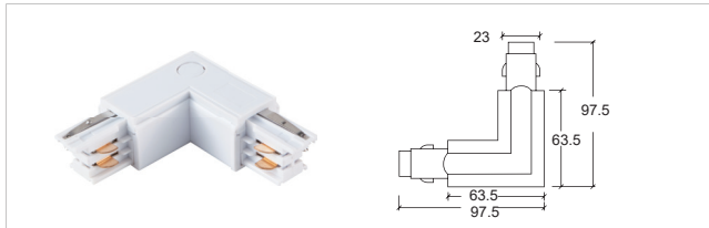
H-04 L型接駁器 - 左 L- connector - L
