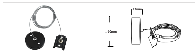
任意角度接驳器 Flexible Connector
