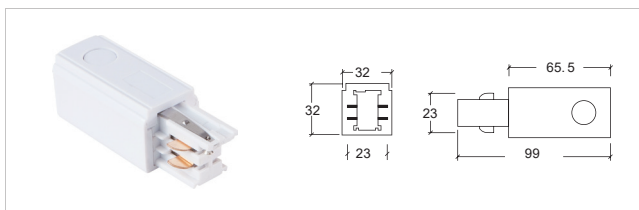
H-04 电源接駁器 - 右 Feeder-R
