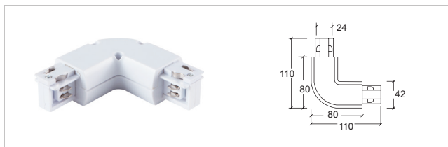
H-01 L型接驳器 - 左 L- connector - L
