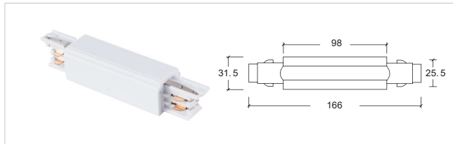
H-04 直线接駁器 Straight connector
