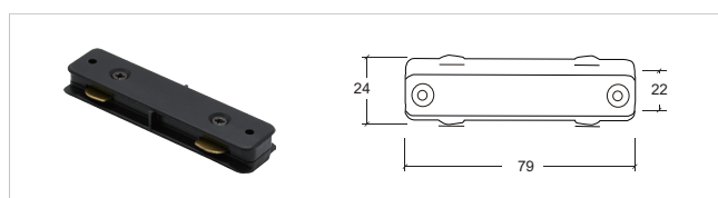
二线桥架外L接L Connector YZ6216-L
