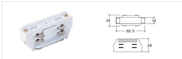
H-01 迷你型直连接驳器 Straight connector MINI I
