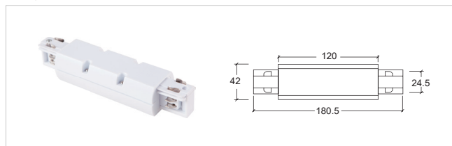
H-01 直连接驳器 Straight connector
