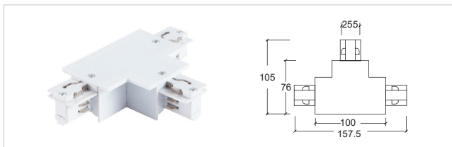
H-03 三向接驳器 - 右 T- connector - R
