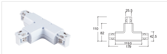
H-01 三向接驳器 - 左 T- connector - L
