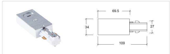
3 线 A 电源接驳器 - 右 Feeder-R
