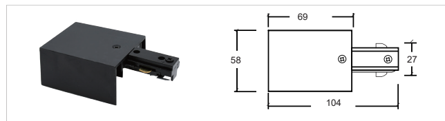
桥架吊装件 Track Rail Suspending YZ6222/6317-D
