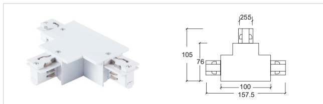
H-03 三向接驳器 - 左 T- connector - L
