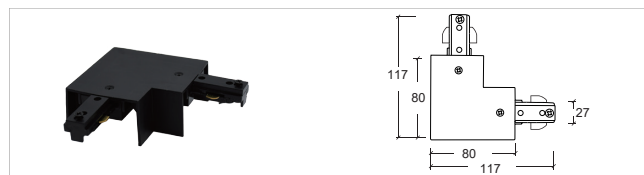
三线桥架外X接X Connector YZ6317-T
