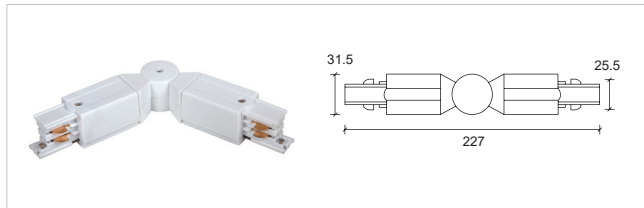
H-04 任意角度接駁器 Flexible Connector
