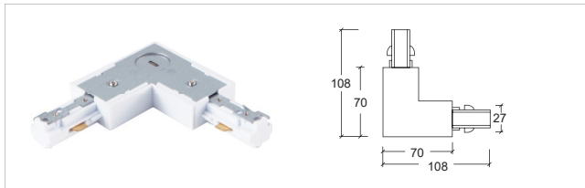
3 线 A L 型接驳器 - 右 L-connector - R
