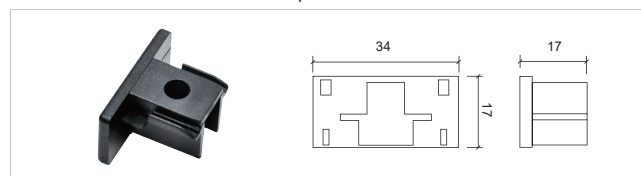
3 线 A 直线接驳器 YZ6313- I Connector
