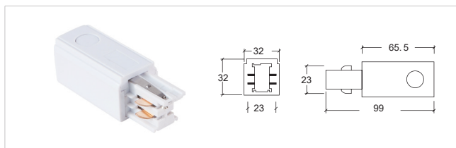
H-04 电源接駁器 - 左 Feeder-L
