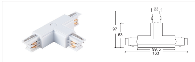
H-04 三向接駁器 - 右 T- connector - R
