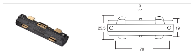
三线桥架外L接L Connector YZ6306-L
