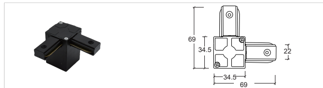
二线桥架外T接T Connector YZ6216-T
