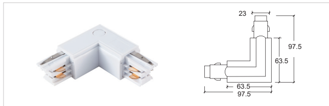
H-04 L型接駁器 - 右 L- connector - R
