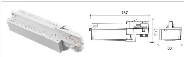
四线长电器箱 Four wire long electrical box S030
