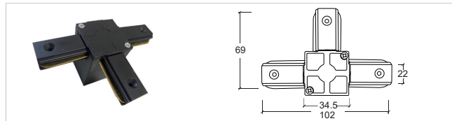
二线桥架外X接T Connector YZ6216-X
