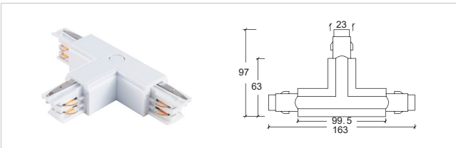
H-04 三向接駁器 - 左 T- connector - L
