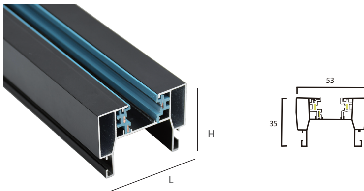
三线桥架电源头前插 feeder YZ6309-Q
