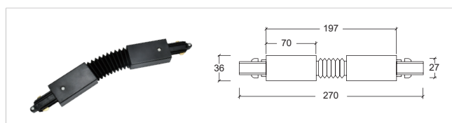
3 线 A 多角度接驳器 (软接) YZ6313-Soft Connector
