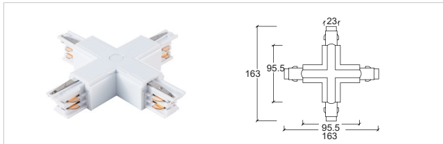
H-04 四向接駁器 X- connector
