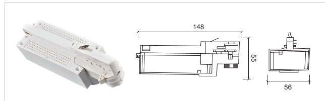
四线迷你小盒 Four - wire mini box S027
